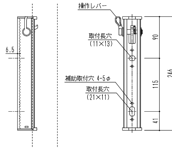
取付ブラケット詳細図
